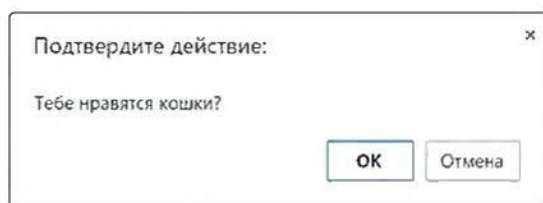
Рис. 7.2. Диалог confirm
