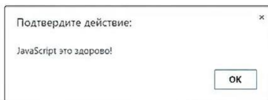
Рис. 7.3. Диалог alert
