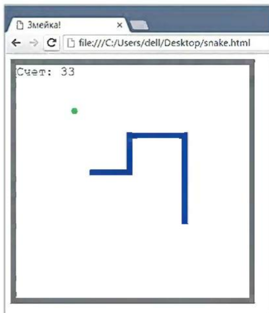
Рис. 16.1. Наша «Змейка»
